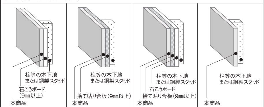
下地条件(壁、天井施工共通)
