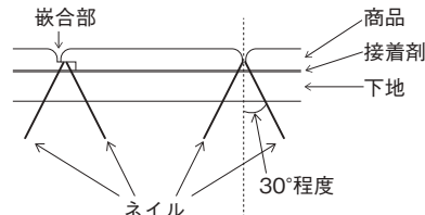
【ネイルでの固定概要図】
