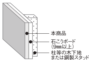
【下地が石こうボードのみの例】
