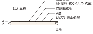
■ 断面図
