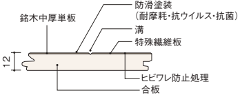
■ 断面図
